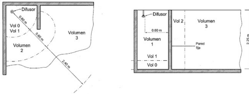
Figura 6 – DUCHA SIN PLATO PERO CON PARED FIJA. DIFUSOR FIJO
