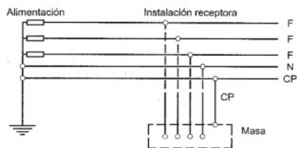
Figura 1. Esquema de distribución tipo TN-S
