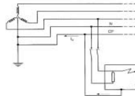
Figura 3. Esquema TN-S.
