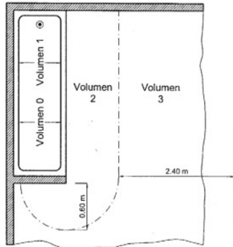
Figura 2 – BAÑERA CON PARED FIJA
